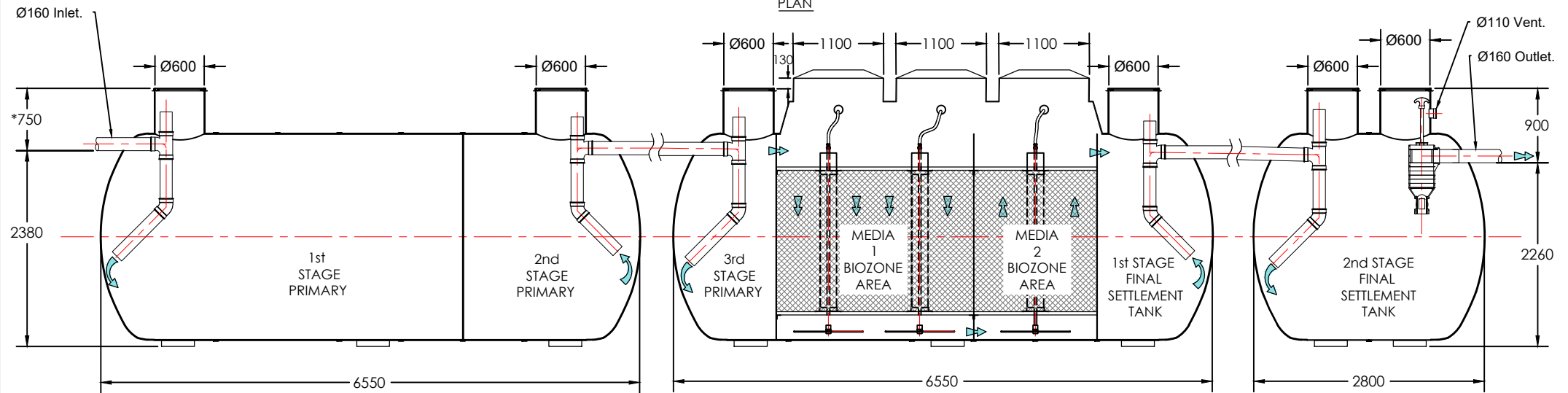
SECTION A-A
