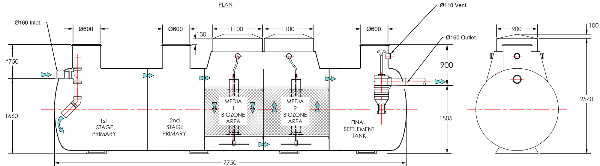
SECTION A-A
